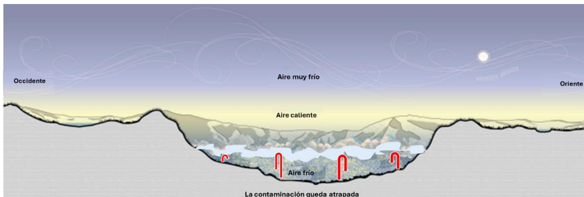
Figura 60 Fenómeno de inversión térmica (Área Metropolitana del Valle de Aburrá y Universidad EAFIT, 2019).
